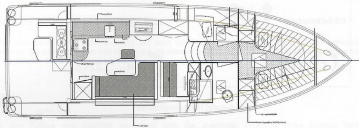
Figur: Generalplan
