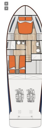
AP 44 Sedan layout
